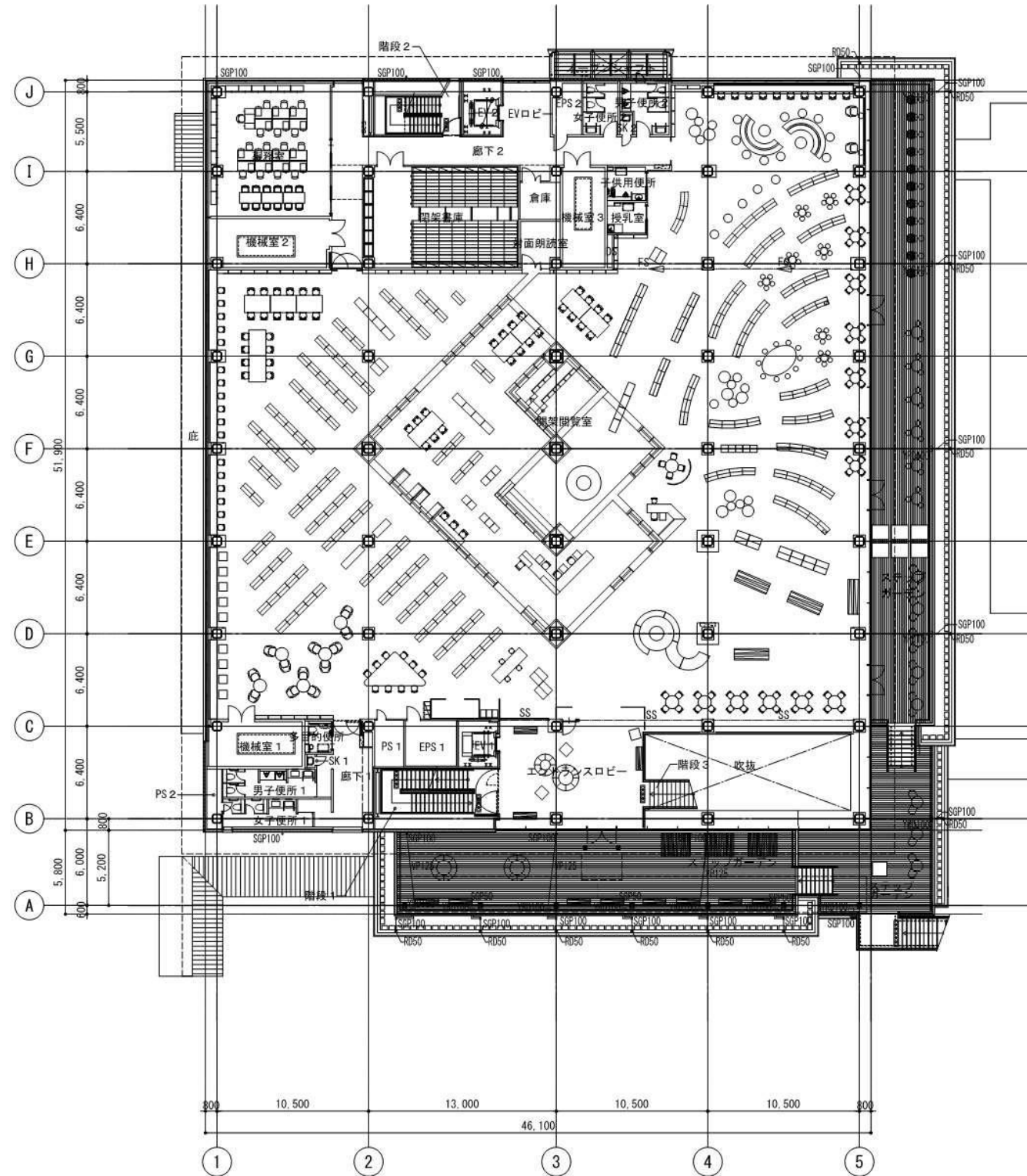
2階平面図
