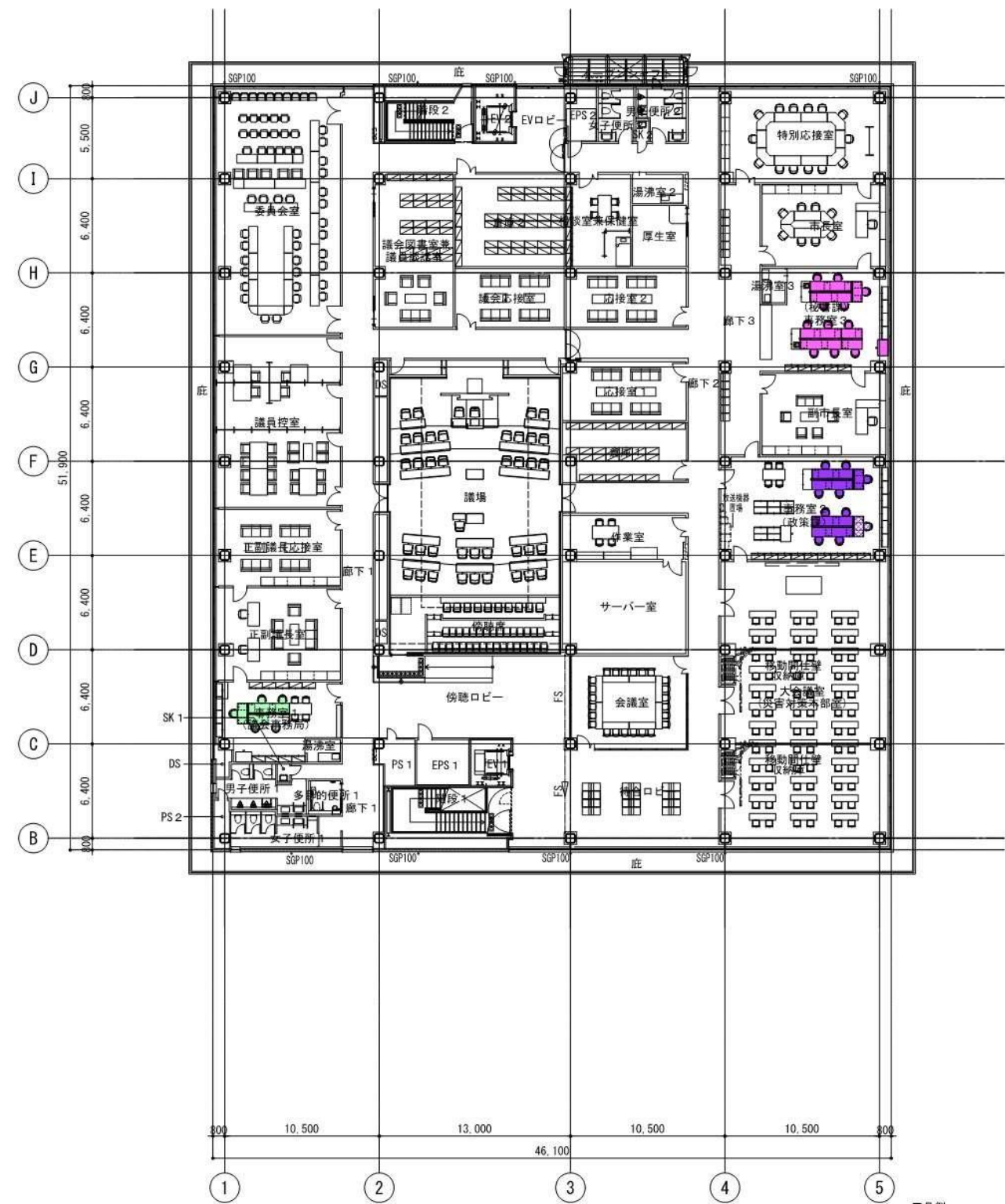
4階平面図
