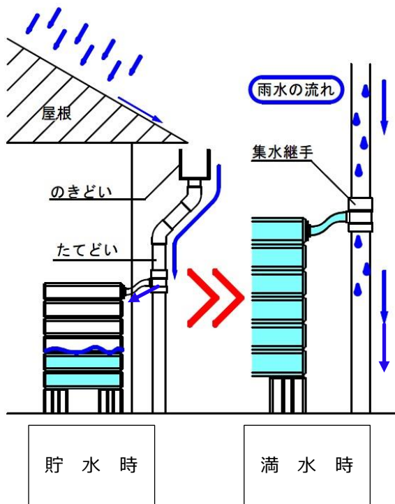
【 雨水が雨水貯留槽に溜まるまでの流れ 】
